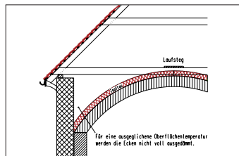
Wärmebrücken vermeiden
