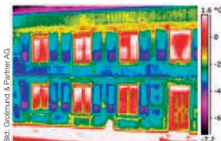
Die Wärmebildkamera zeigt die Isolationschwachpunkte.
